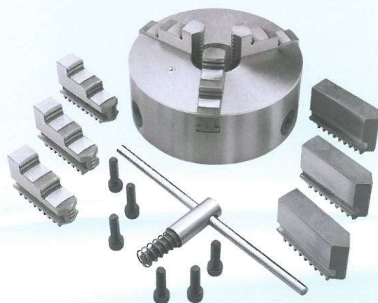
Bucha para torno corpo em ferro fundido com mordentes em aço temperado
